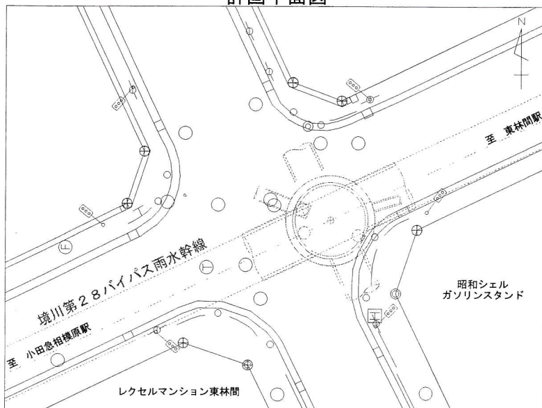
計画平面図
