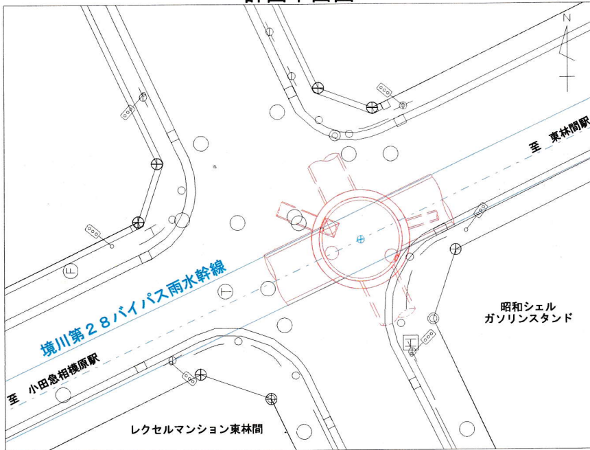
計画平面図
