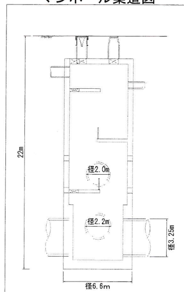
マンホール築造図
