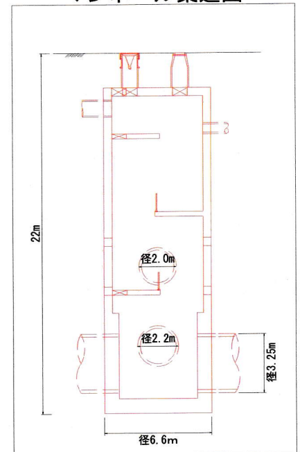
マンホール築造図
